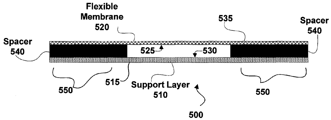
FIG. 5A Membrane Switch (OFF)
