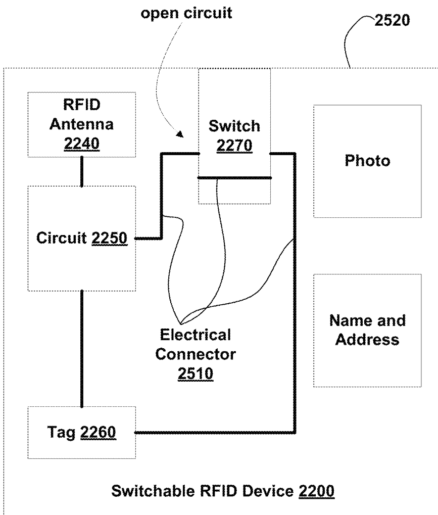
OFF Position FIG. 25A
